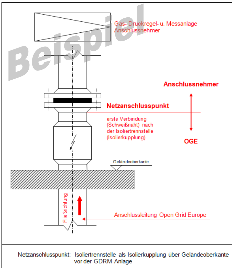
Abbildung 6: Prinzipskizze
