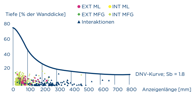
Molchanzeigentiefe und -länge mit DNV-Grenzkurve
